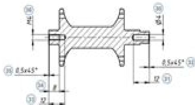
A-A (1:1)
